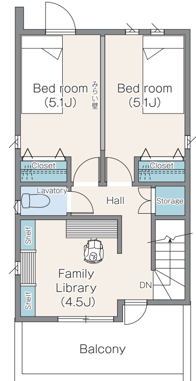
3F
